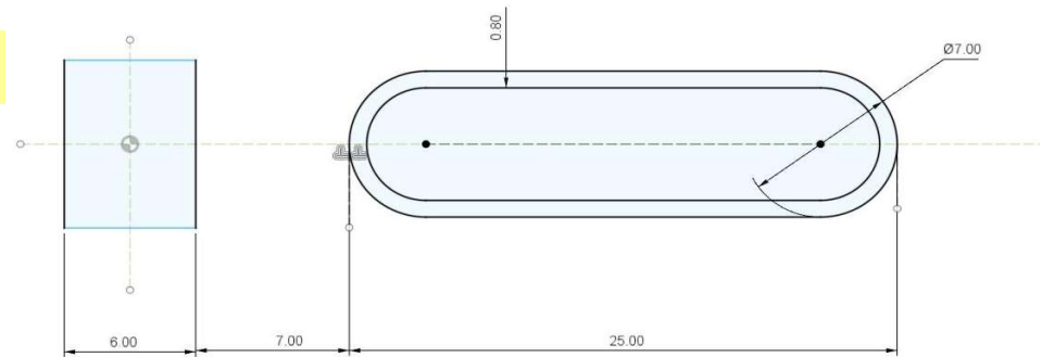
Aussparung für HLW-Kabel/Stecker in Seitenflosse
